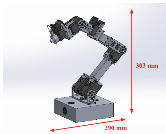
Fig. 4-4 共通マニピュレータ (SolidWorks)
