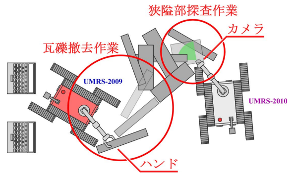
Fig. 2-8 エンドエフェクタの取替え
