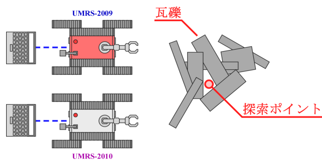
Fig. 2-4 モバイルロボットの協調作業
