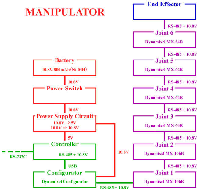
Fig. 4-5 システム構成図
