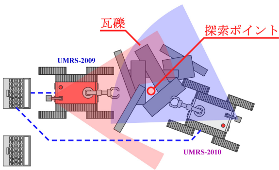
Fig. 2-6 カメラ画像の共有
