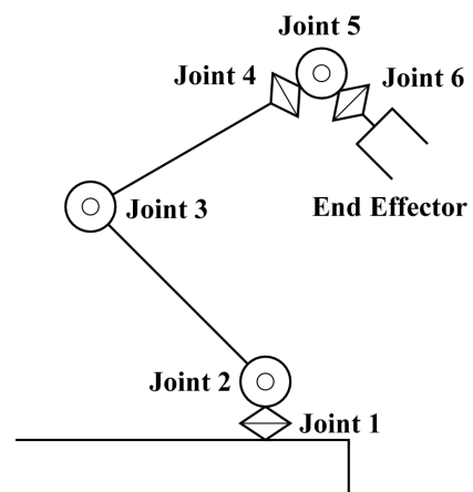
Fig. 4-1 共通マニピュレータのリンク機構
