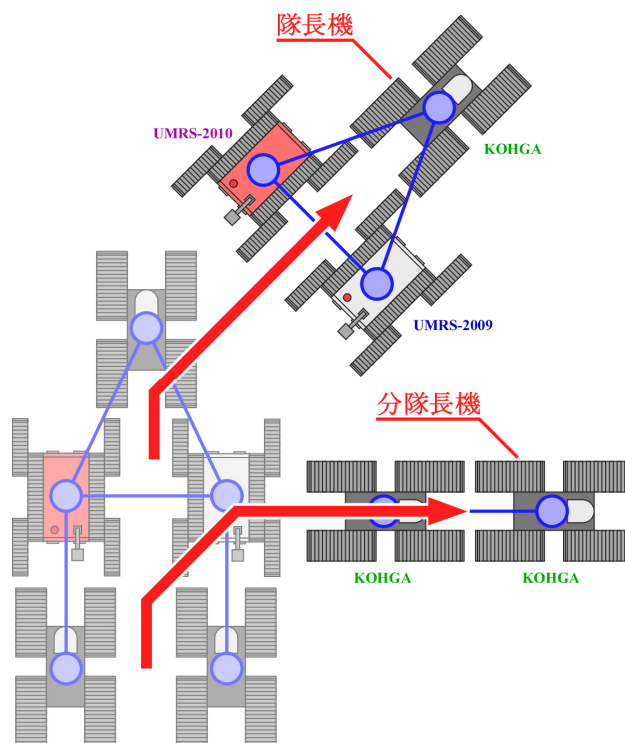
Fig. 2-3 モバイルロボット群の分隊
