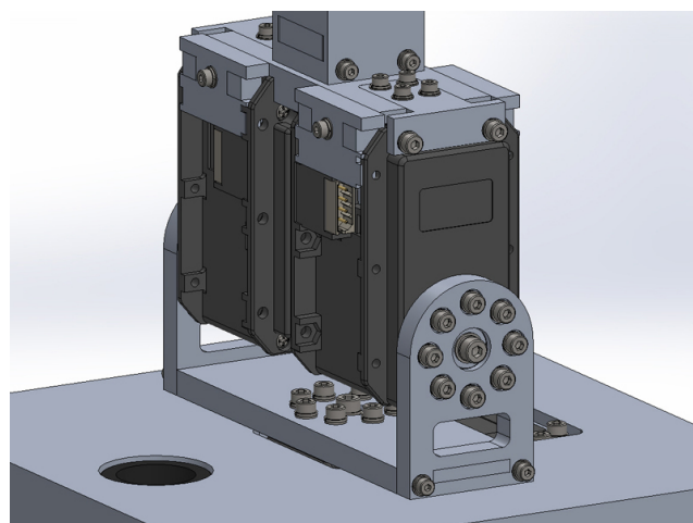
Fig. 4-5 ダブルモータ (SolidWorks)
